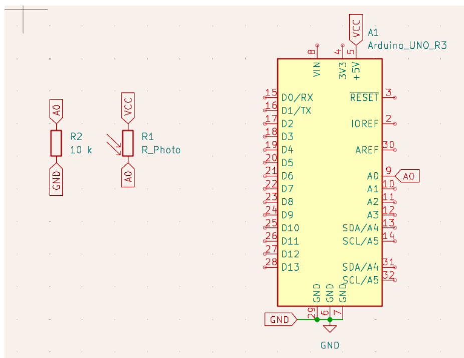
図 19 楽器デバイスの受光部の回路図
